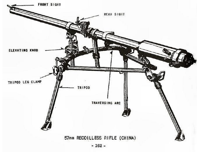
Figura 4: Cañón sin retroceso de 57 mm
